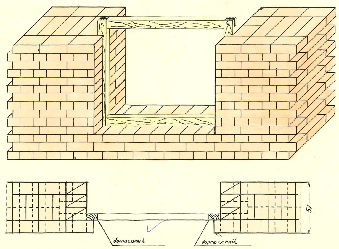
pogled špalete sa doprozornikom
