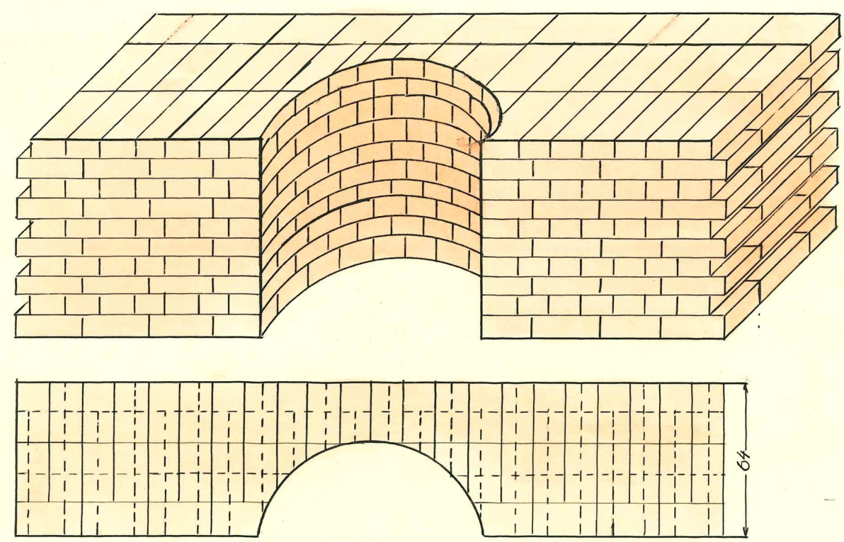
pogled zidne udubine
