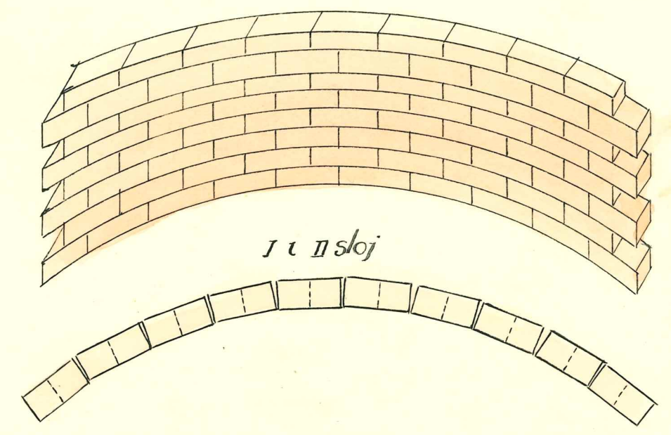
pogled okruglog zida
