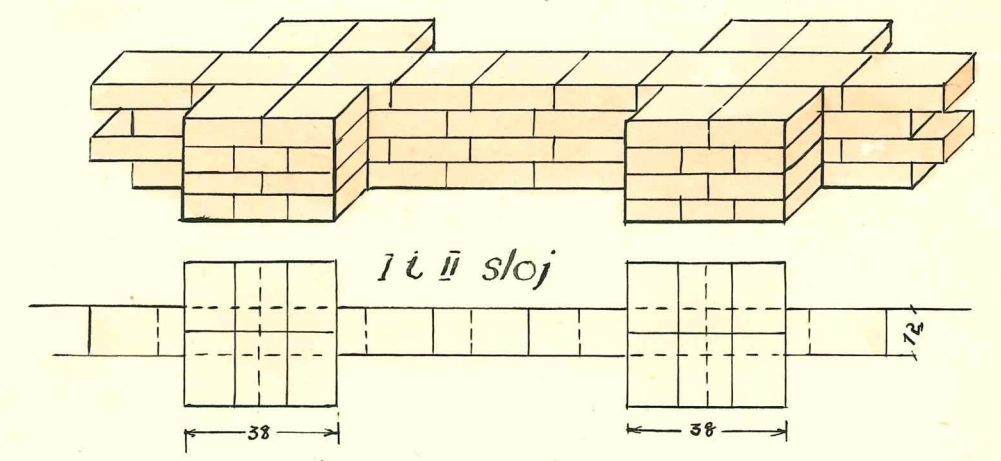
pogled zidnog istaka 1/4 opeke
