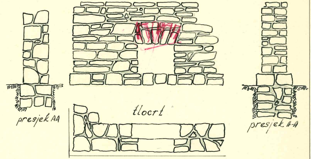
zid od grubo obradenog lomljenog kamena
