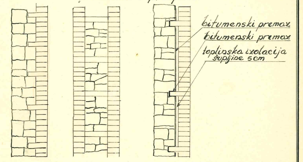
Načini obloženja kamenog zida opekama prikazano u presjeku
