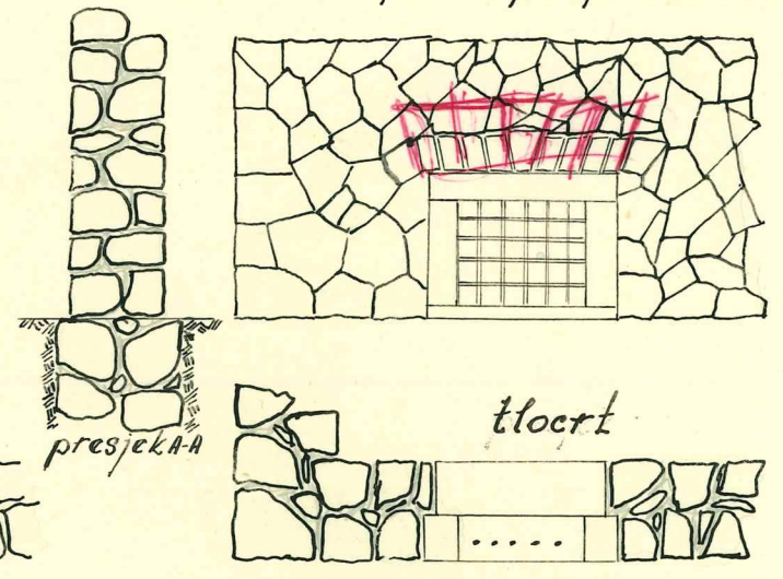
ciklopski ili poligonalni zid
