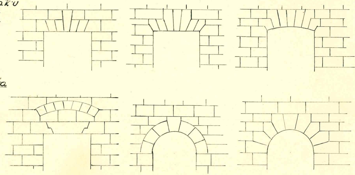
Oblici lukova od naravnog kamena
