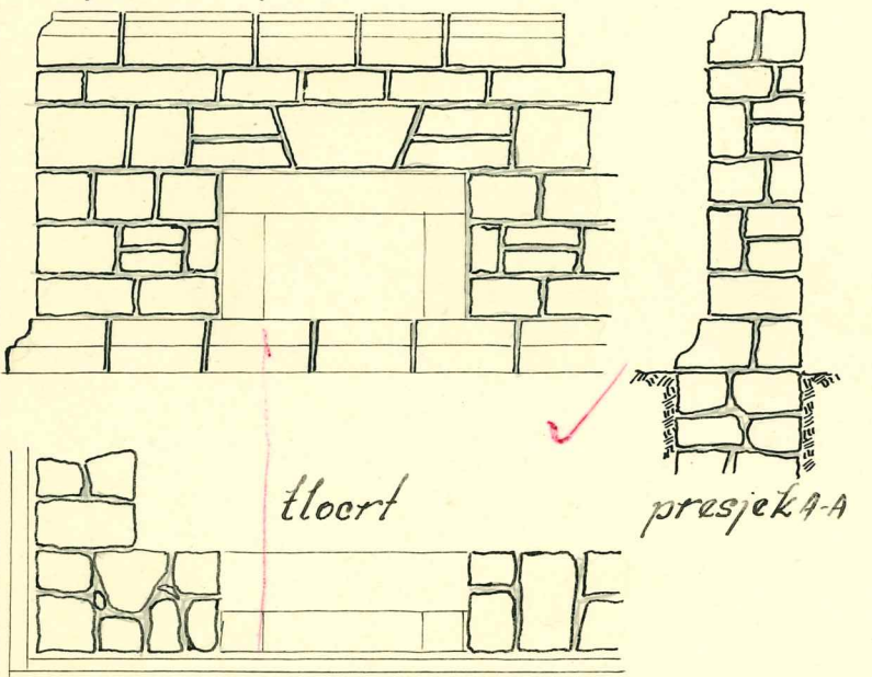
oploćenje kamenim pločama
