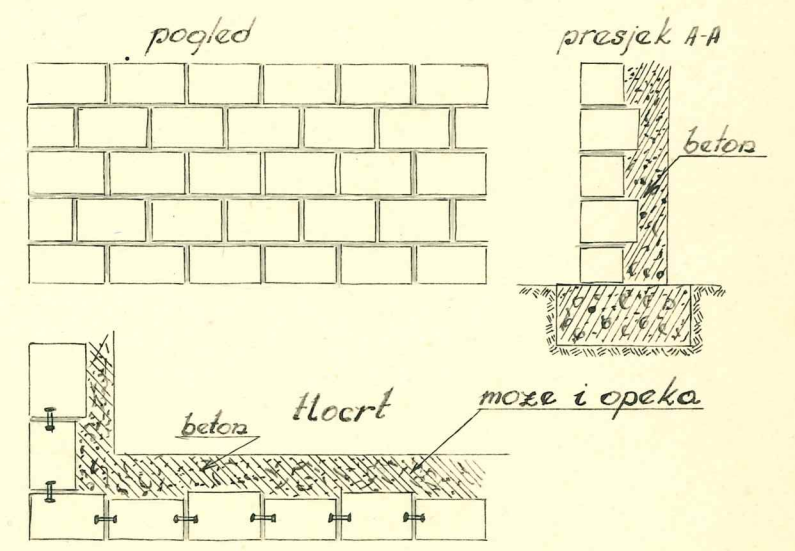
1/2ješoviti zid od kamena i betona
