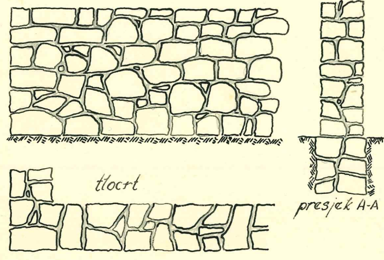
Slojzid od grubo obradenog kamena
