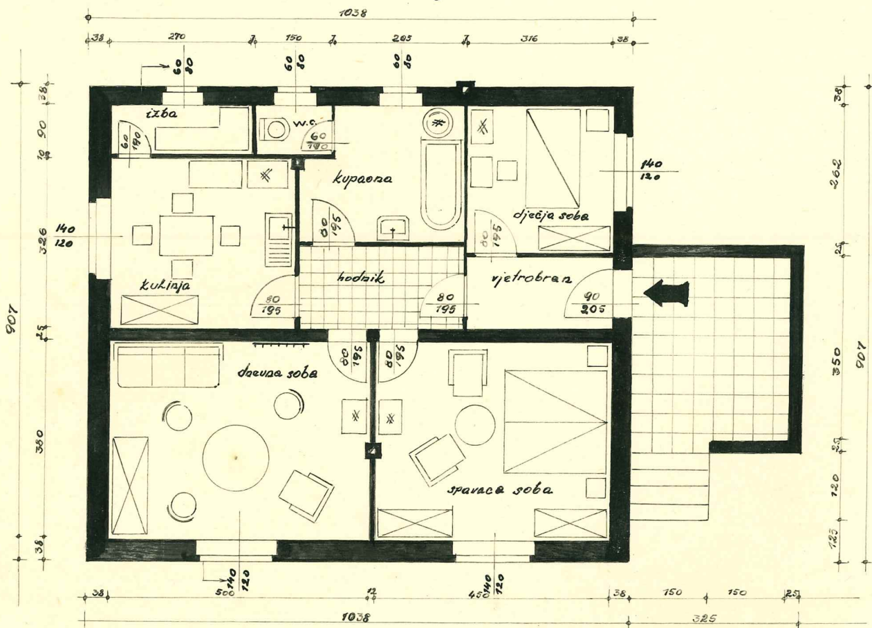
tlocrt prizemlja
