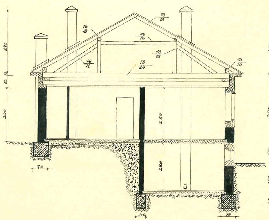
presjek A-A
