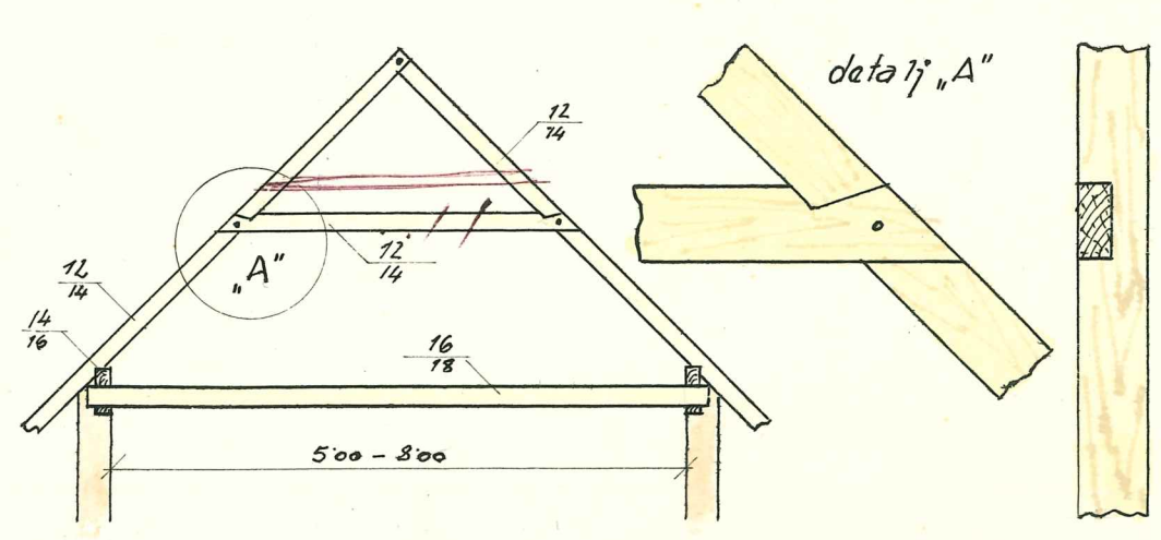
horizontalno rješenje jednostruke stolice
