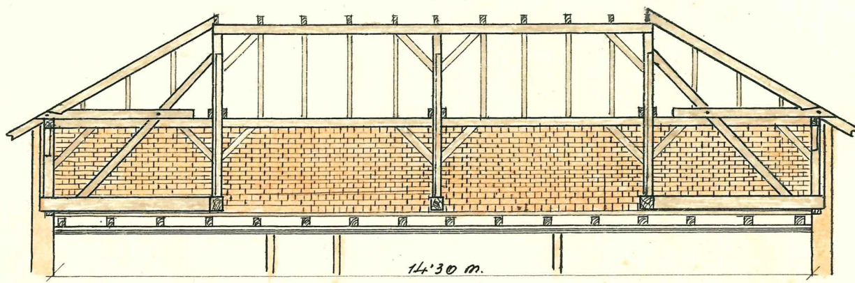
uzdužni presjek.
