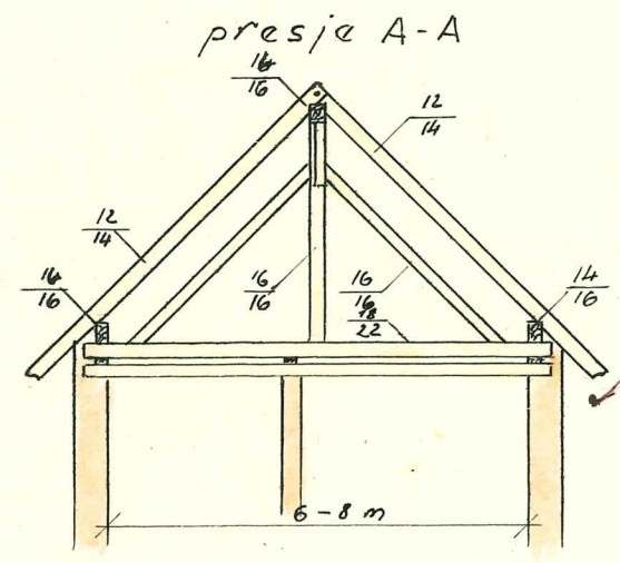
jednostruka stolica sa nedstrešnim zidom presjek
